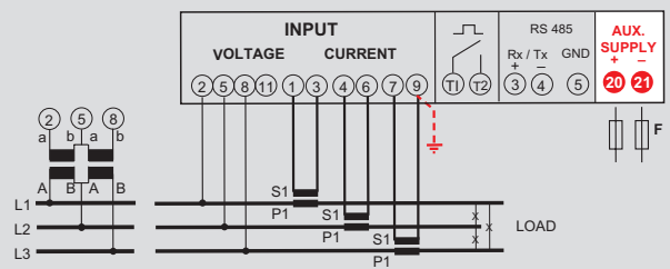
Dreiphasenleitung 3 Leiter
