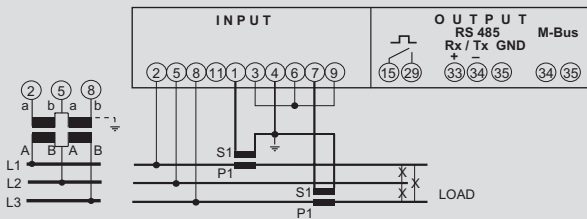
Dreiphasenleitung 3L; ungleich belastet (ARON L1-L3)
