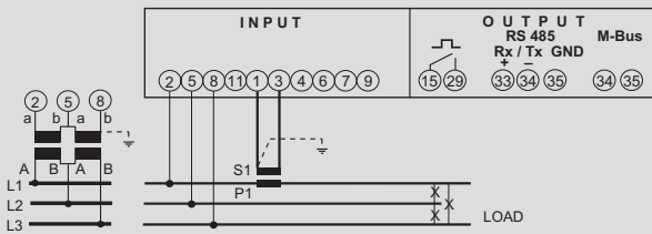
Dreiphasenleitung 3L, gleich belastet
