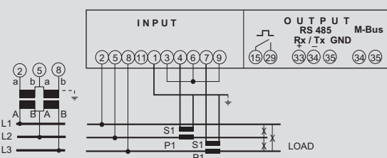
Dreiphasenleitung 3L; ungleich belastet (ARON L2-L3)
