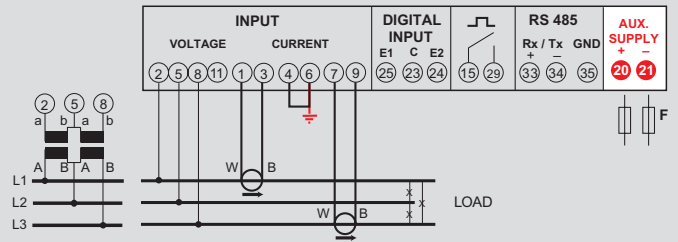
Dreiphasenleitung 3 Leiter (ARON L1-L3)
