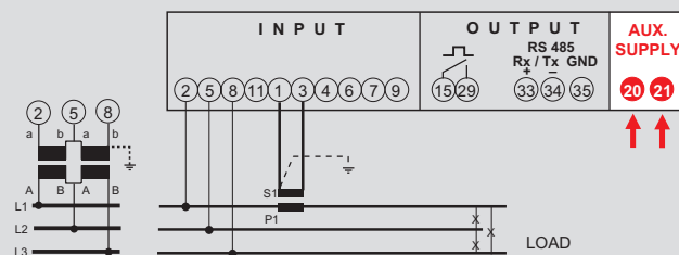
Dreiphasenleitung 3 Leiter, 1 CT
