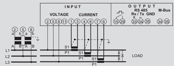
Dreiphasenleitung 3L, ungleich belastet
