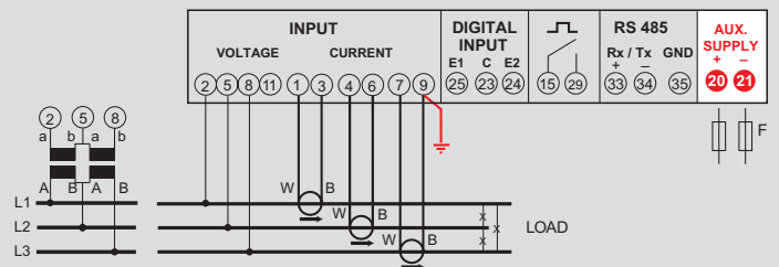
Dreiphasenleitung 3 Leiter
