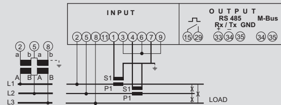
Dreiphasenleitung 3L; ungleich belastet (ARON L1-L2)
