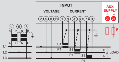
Dreiphasenleitung 3 Leiter
