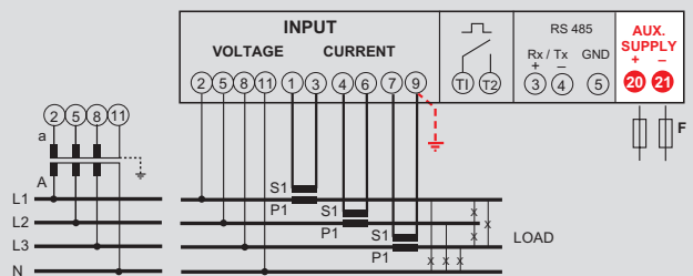
Dreiphasenleitung 4 Leiter
