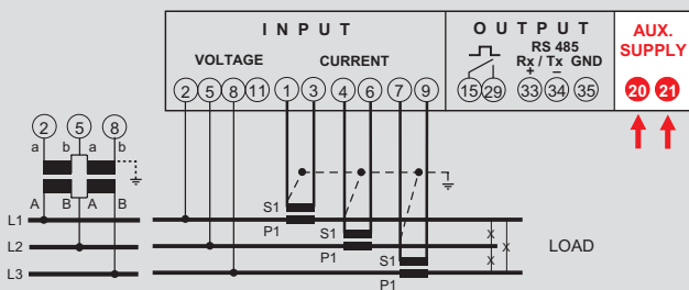
Dreiphasenleitung 3 Leiter
