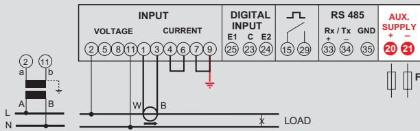
Einphasenleitung
