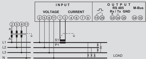
Dreiphasenleitung 3P + N, gleich belastet
