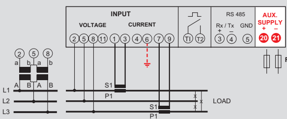
Dreiphasenleitung 4 Leiter (ARON L1-L3)
