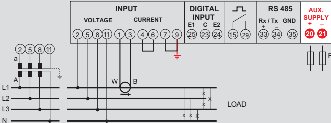
Dreiphasenleitung 4 Leiter, 1 CT
