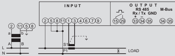
Einphasenleitung
