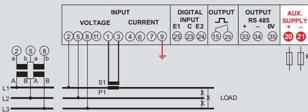
Dreiphasenleitung 3 Leiter, 1 CT
