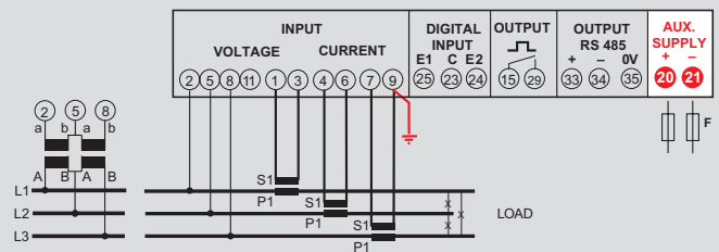
Dreiphasenleitung 3 Leiter
