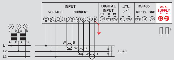
Dreiphasenleitung 3 Leiter
