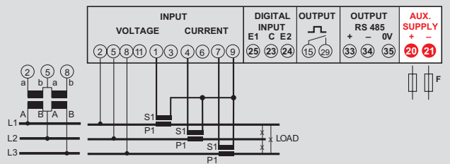
Dreiphasenleitung 3 Leiter
