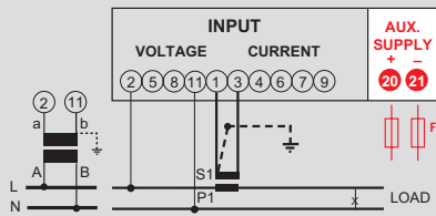
Einphasenleitung
