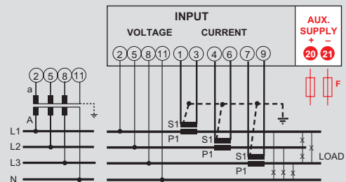
Dreiphasenleitung 4 Leiter
