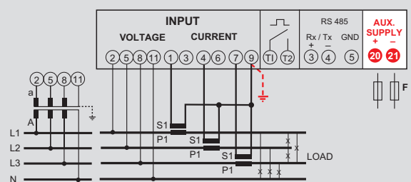
Dreiphasenleitung 4 Leiter
