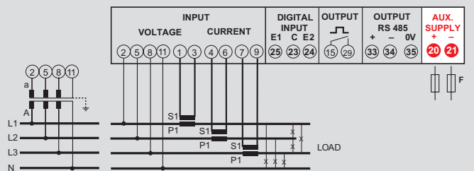
Dreiphasenleitung 4 Leiter
