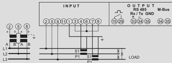
Dreiphasenleitung 3L; ungleich belastet (ARON L2-L3)
