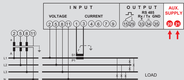
Dreiphasenleitung 4 Leiter, 1 CT
