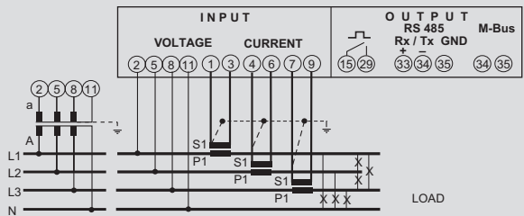
Dreiphasenleitung 3P + N, ungleich belastet
