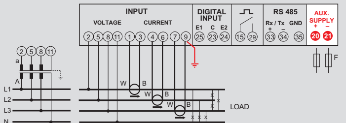
Dreiphasenleitung 4 Leiter
