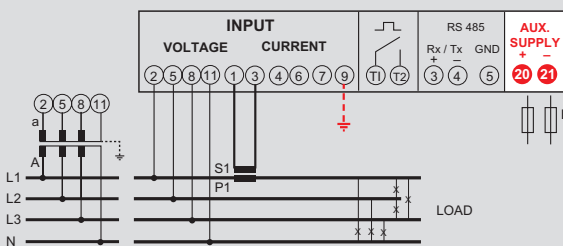
Dreiphasenleitung 4 Leiter, 1 CT
