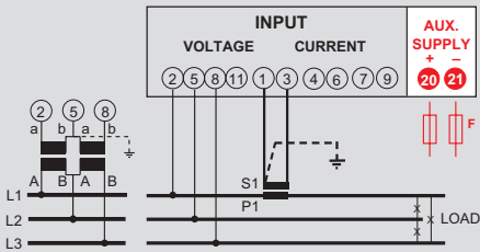
Dreiphasenleitung 3 Leiter, 1 CT
