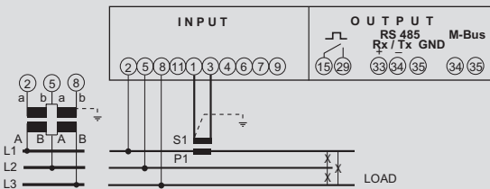
Dreiphasenleitung 3L, gleich belastet
