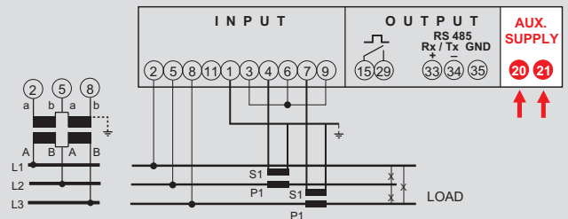
Dreiphasenleitung 3 Leiter (ARON L2-L3)
