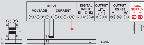
Einphasenleitung
