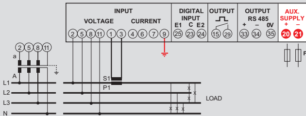
Dreiphasenleitung 4 Leiter, 1 CT
