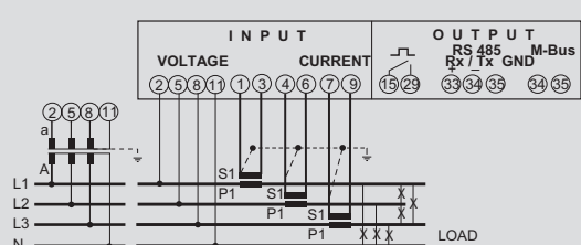
Dreiphasenleitung 3L+N, ungleich belastet
