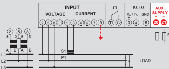
Dreiphasenleitung 3 Leiter, 1 CT
