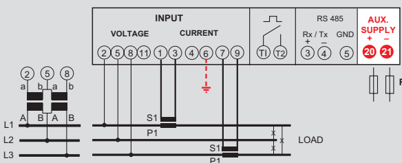
Dreiphasenleitung 4 Leiter (ARON L1-L3)
