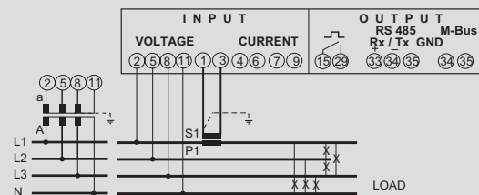
Dreiphasenleitung 3L+N, gleich belastet
