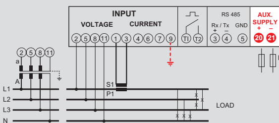
Dreiphasenleitung 4 Leiter, 1 CT
