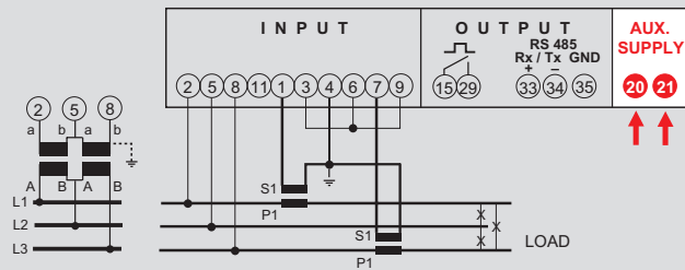
Dreiphasenleitung 3 Leiter (ARON L1-L3)
