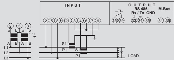
Dreiphasenleitung 3L; ungleich belastet (ARON L1-L2)
