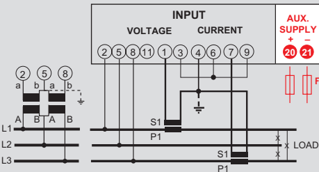
Dreiphasenleitung 4 Leiter (ARON L1-L3)
