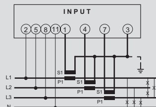
Dreiphasenleitung 4 Leiter
