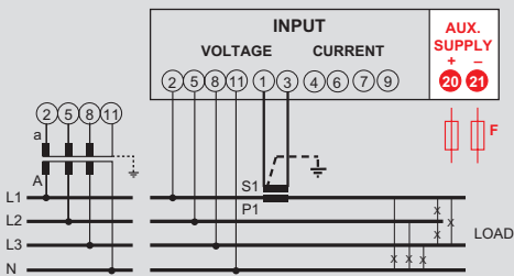
Dreiphasenleitung 4 Leiter, 1 CT
