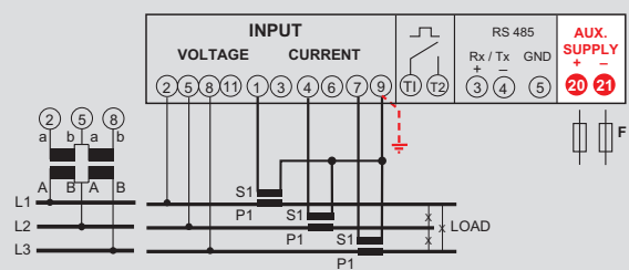
Dreiphasenleitung 3 Leiter
