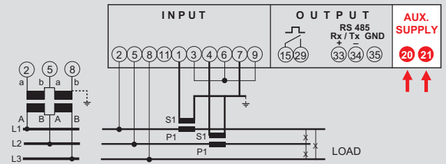
Dreiphasenleitung 3 Leiter (ARON L1-L2)
