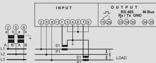
Dreiphasenleitung 3L; ungleich belastet (ARON L1-L3)
