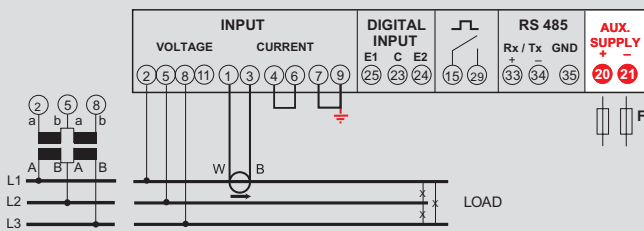
Dreiphasenleitung 3 Leiter, 1 CT
