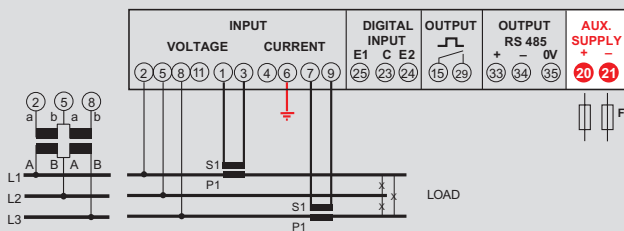
Dreiphasenleitung 3 Leiter (ARON L1-L3)
