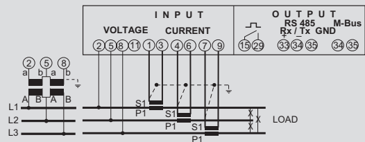
Dreiphasenleitung 3L, ungleich belastet
