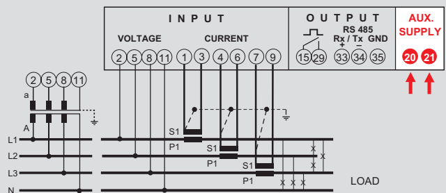
Dreiphasenleitung 4 Leiter
