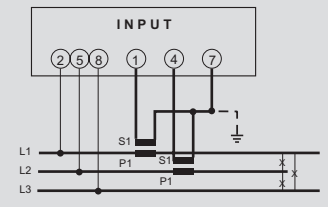
Dreiphasenleitung 3 Leiter (ARON L1-L2)
