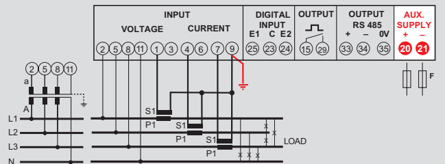
Dreiphasenleitung 4 Leiter
